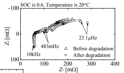
劣化前後の交流インピーダンスと起電力の測定結果
