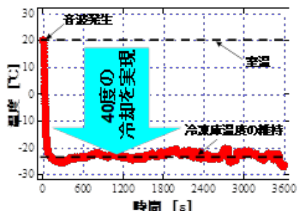
熱音響冷却システムの冷却特性
