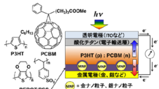
図2 金属ナノ粒子を組み込んだ有機薄膜太陽電池
