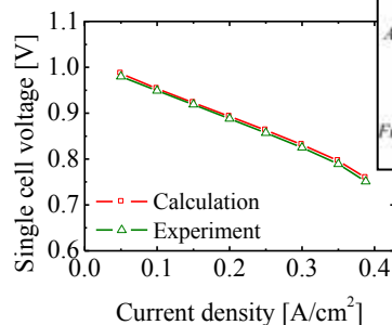
固体酸化燃料電池の解析例（解析モデルと電流－電圧特性）
