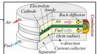
固体酸化燃料電池の解析例（解析モデルと電流－電圧特性）
